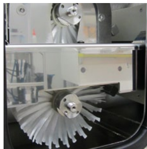
毛刷清洁
