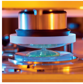
紫外线固化粘合剂保护镜片前表面, 无需使用胶带
