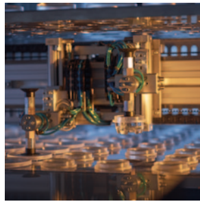
真空操作吸盘拣取盘片
